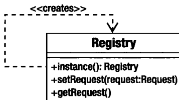
图12-2 一个简单的注册表
