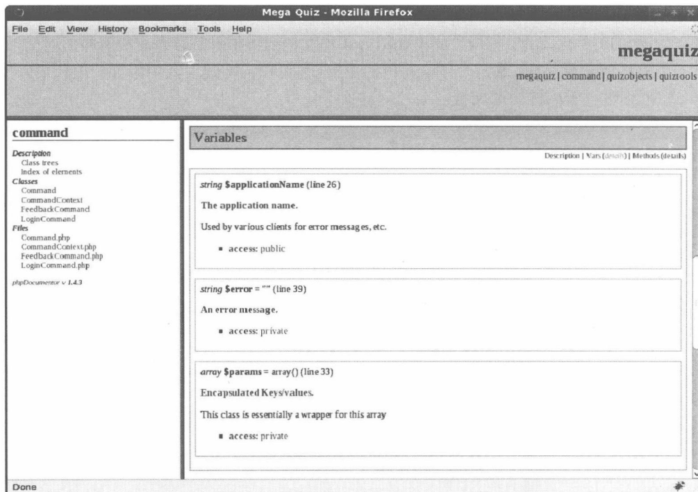
图16-5 属性的文档
