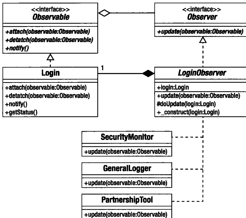
图11-6 观察者模式
