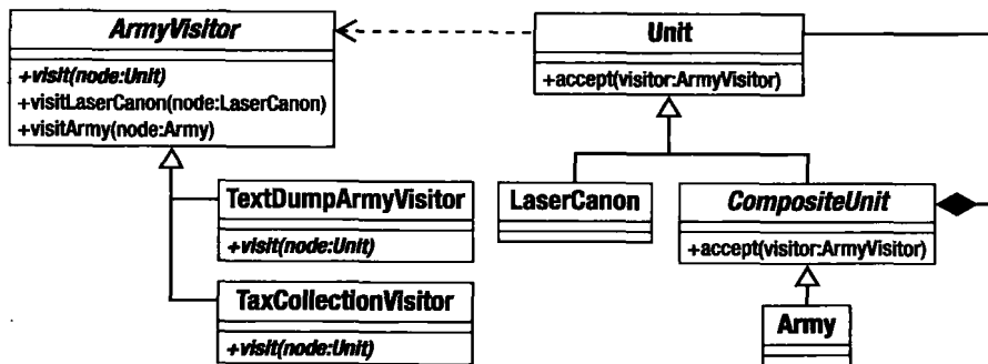
图11-7 访问者模式
