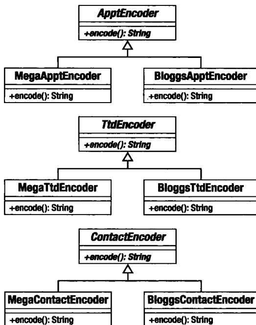
图9-6 产品家族
