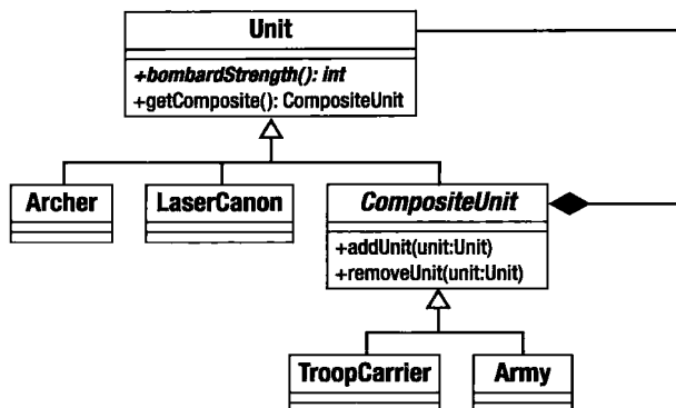
图10-2 从基类中移走add/remove方法
