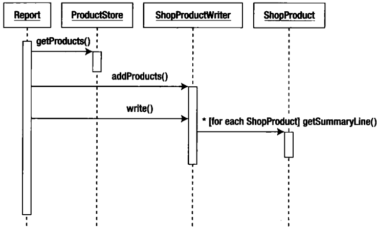
图6-20 完整的时序图
