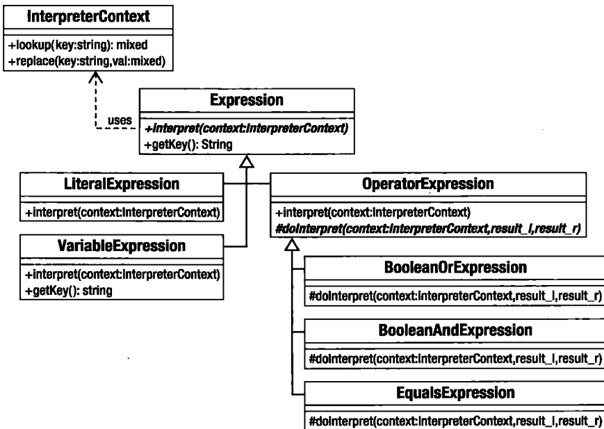
图11-2 解释器模式
