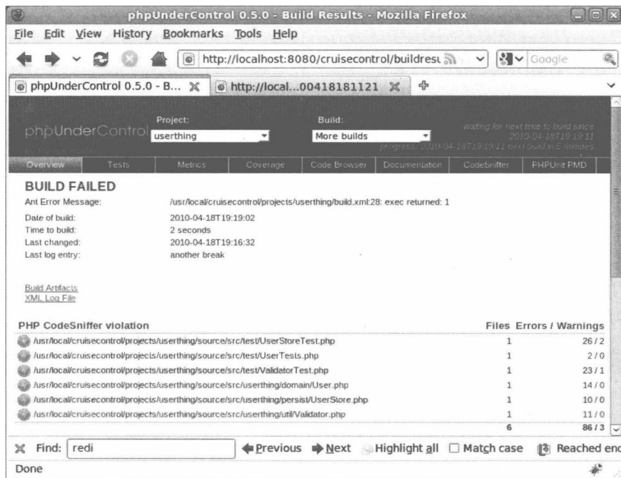
图20-10 构建失败
